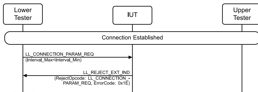
Figure 4.3-257: Reject Invalid Connection Parameter Request Parameters MSC
