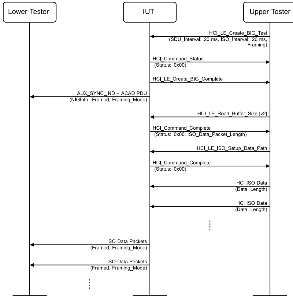
Figure 4.11-13: LE Create BIG Test Framing Parameter MSC
